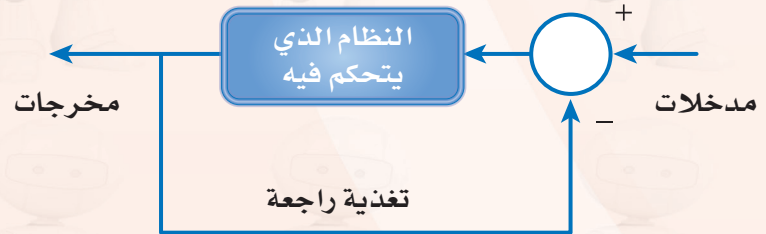
شكل (٤-٨): المكونات الرئيسية في نظام التحكم ذي الدائرة المغلقة
