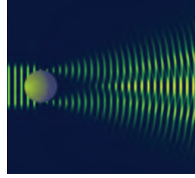
الشكل ٩ يعتمد حيود الموجة وانعاطفها حول الجسم على حجم (أبعاد) الجسم وعلى طول الموجة.
