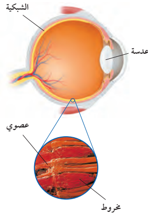
الشكل ٢٤ الخلايا المخروطية والعصوية في شبكة العين تُحدّد الضوء، وترسل إشارات عصبية للدماغ.
