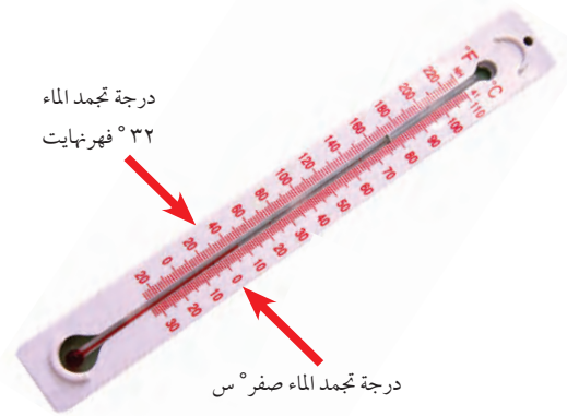
الشكل ٢ تستخدم مقاييس الحرارة الشائعة ومنها المقياس السيليزي والمقياس الفهرنهايتي في قياس درجة الحرارة.
