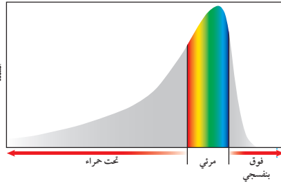
موجات كهرومغناطيسية من الشمس
