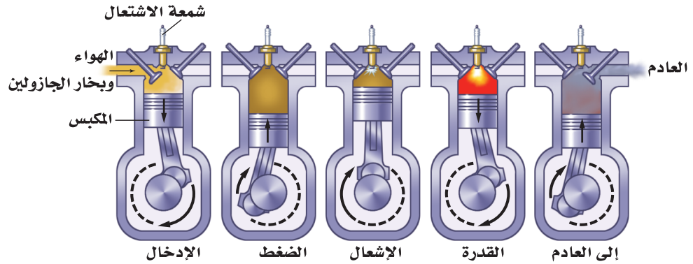
■ الشكل 6-12 تعمل الحرارة الناتجة بفعل احتراق الجازولين على تمدد الغازات الناتجة وبذل قوة وشغل على المكبس.
