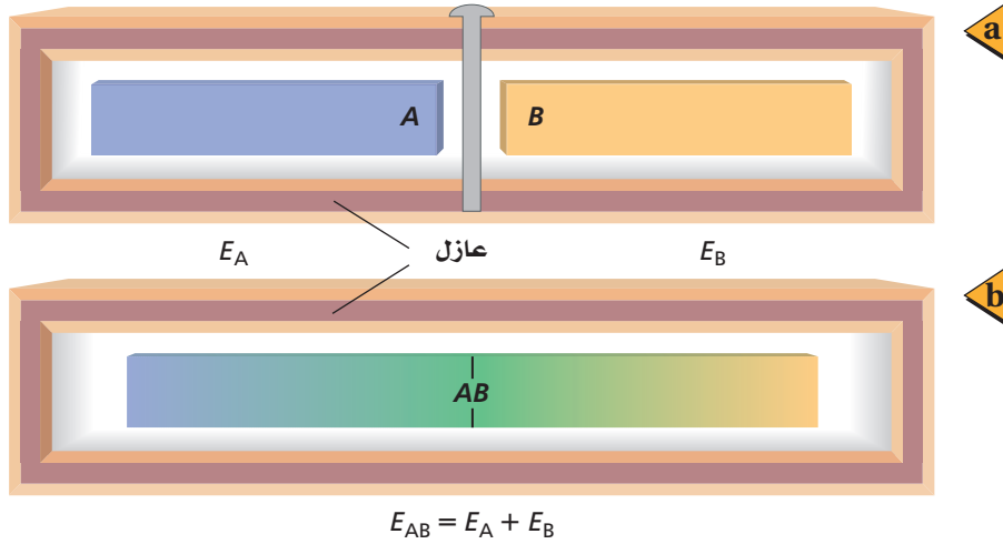
■ الشكل 8-6 نظام مكون من نموذجين لـ قالبين عند درجات حرارة مختلفة، وهما مفصولان في الحالة الابتدائية (a). وعندما يتلامس القالبان فإن الحرارة تتدفق من القالب الساخن إلى القالب الأبرد (b). وتبقى الطاقة الكلية ثابتة.
