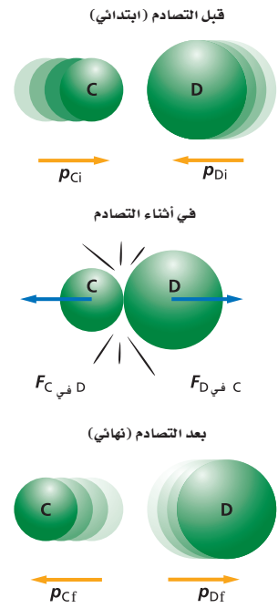
■ الشكل 3-4 عندما تصطدم كرتان فإن كلا منهما تؤثر في الأخرى بقوة مما يؤدي إلى تغير زخميهما.
