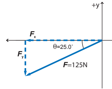
■ الشكل 3-4 إذا أثرت قوة في مركبة بزاوية، فإن القوة المحصلة التي تبذل الشغل هي مركبة القوة التي تؤثر في اتجاه إزاحة الجسم.
