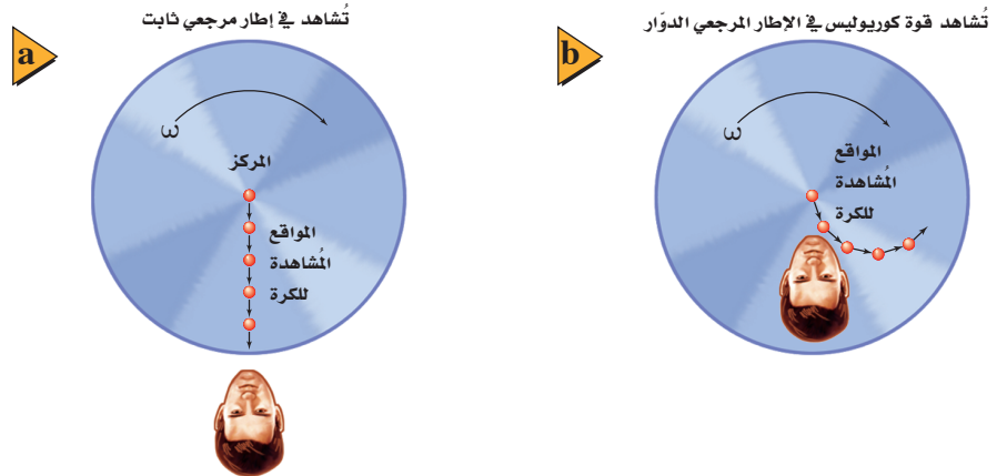
الشكل 2-12 قوة كوريوليس توجد فقط في الأطر المرجعية الدوارة.
