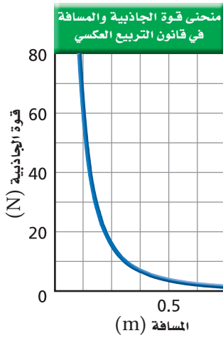
■ الشكل 1-4 تتغير قوة الجاذبية بتغير المسافة وفق قانون التربيع العكسي.
