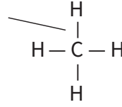
الصيغة البنائية
