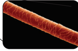
الشكل 3-8 يتكون شعر الإنسان من بروتين ليفي يسمى الكيراتين.
