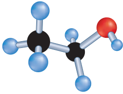
إيثانول
