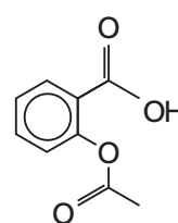
a. حمض الأسيتيل ساليسيليك
