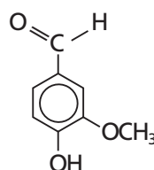
b. الفانيلين
