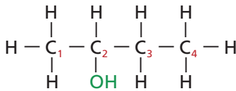
2. b - بيوتانول
