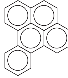
بنزوباييرين
