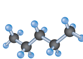
بنتان درجة الغليان = 36^{\circ}C
