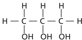
d. 1، 2، 3-بروبان ترايول (الجليسرول)
