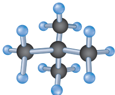
-2،2-ثنائي ميثيل بروبان درجة الغليان = 9^{\circ}C
