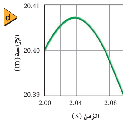
■ الشكل 15-3 في نظام إحداثي اتجاهه الموجب إلى أعلى: a و b تتناقص سرعة الكرة المقذوفة إلى أعلى حتى تصبح صفراً بعد زمن 2.04 s ثم تزداد سرعتها في الاتجاه السالب في أثناء سقوطها. c و d يُظهر الرسمان البيانيان لمنحنى (الإزاحة - الزمن) ارتفاع الكرة في فترات زمنية مماثلة.
