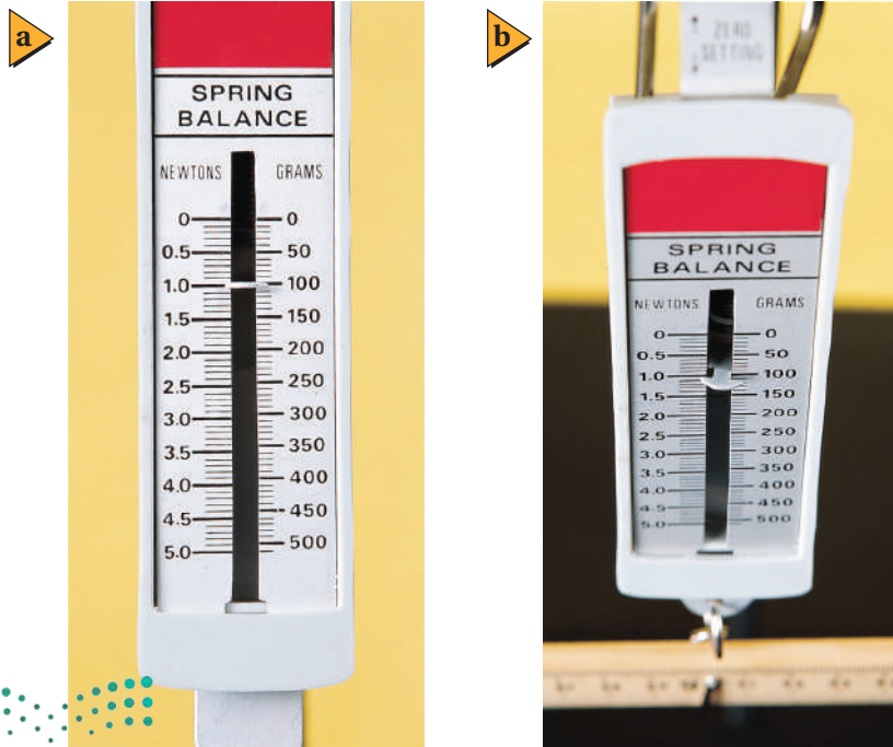
■ الشكل 12-1 عند النظر إلى التدريج بشكل عمودي كما في (a) تكون قراءة تلك أضبط مما لو نظرت بشكل مائل كما في (b).
