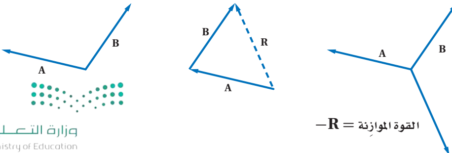
الشكل 12-5 للقوة الموازنة مقدار القوة المحصلة نفسها، ولكنها تعاكسها في الاتجاه.
