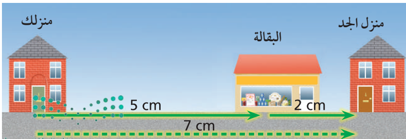
■ الشكل 8-2 يُجمع متجهان بوضع رأس الأول ملائماً لذيل الثاني. تبدأ المحصلة من ذيل المتجه الأول وتنتهي عند رأس المتجه الثاني.
